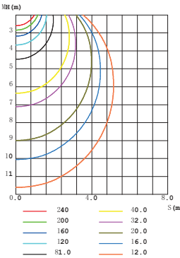
室内灯具配光曲线
