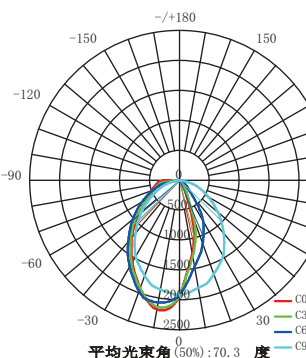
室内灯具配光曲线
